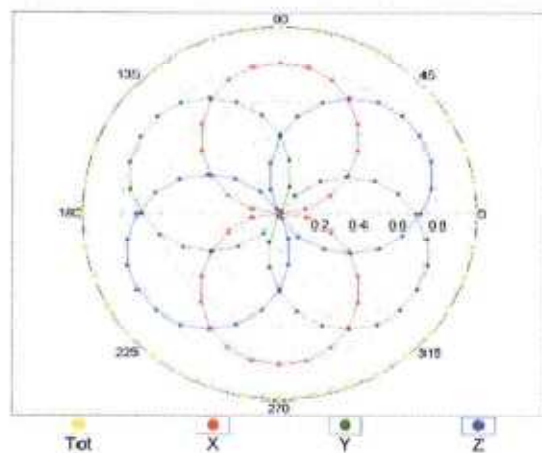
f=1800 MHz,R22
