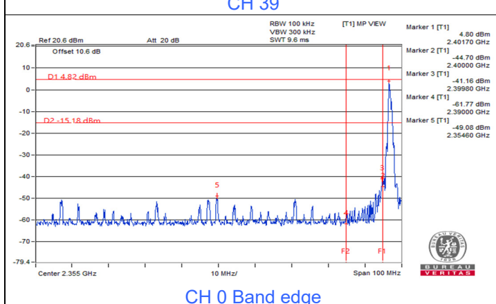
CH 0 Band edge
