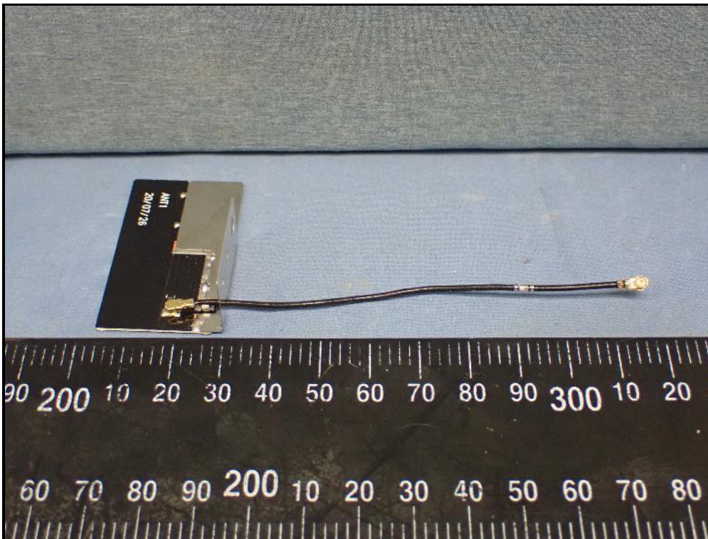
ANT 0 (Brand: FIH / Model: PCB)
