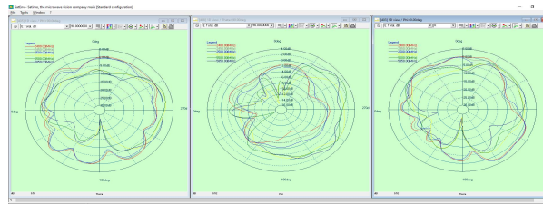
FPC天线 天线形式：IFA天线
