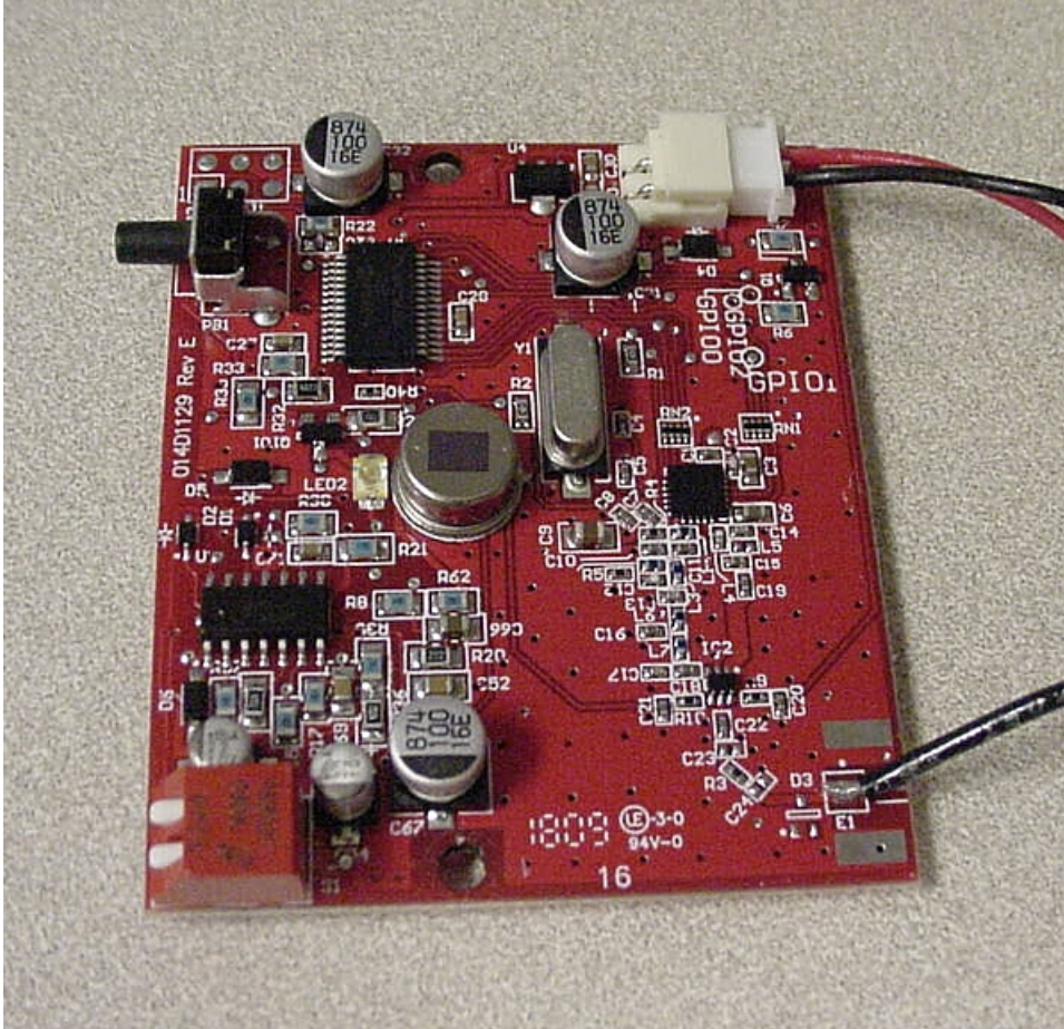
Top PCB
