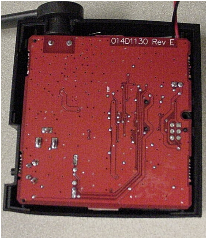
PCB - Bottom
