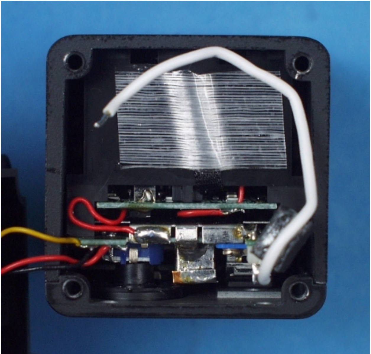
Antenna
