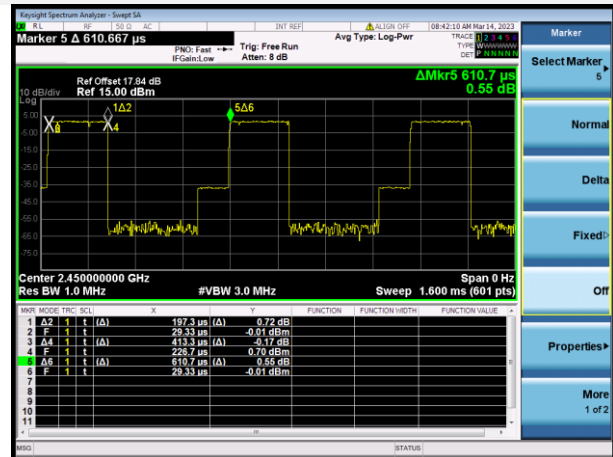
FSK(2Mbps)
