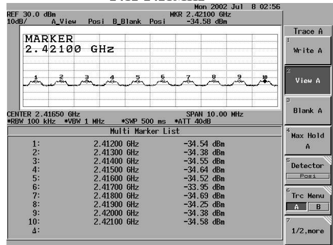
2412-2421MHz
