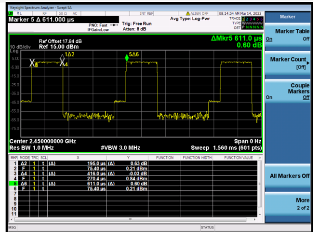
FSK(2Mbps)
