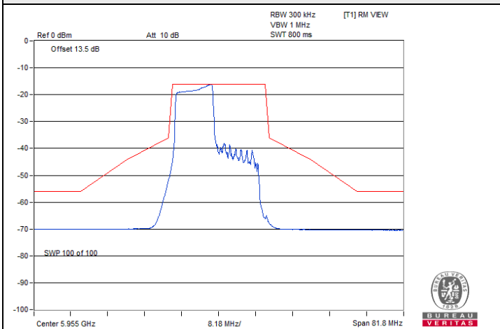
802.11be (EHT20) 106-tone RU / Chain 1 : CH 1@53
