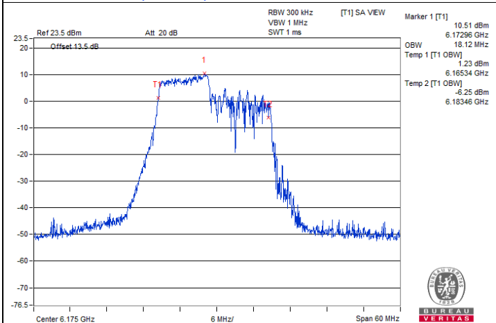
802.11be (EHT20) 106-tone RU / Chain 1 : CH 45@53
