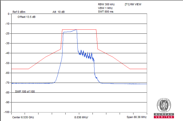
802.11be (EHT20) 106-tone RU / Chain 0 : CH 117@53
