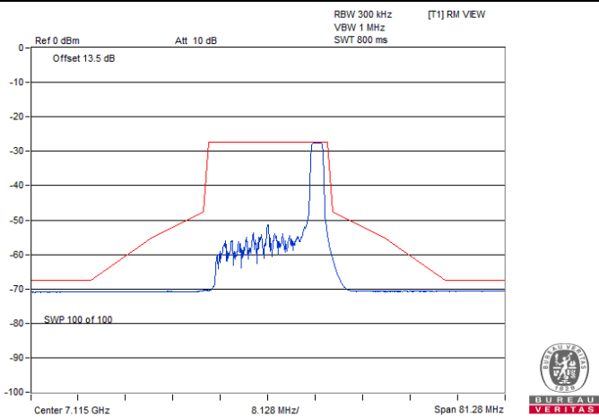
802.11be (EHT20) 26-tone RU / Chain 0 : CH 233@8
