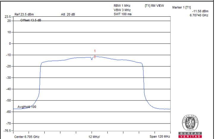
802.11be (EHT80) 996-tone RU / Chain 1 : CH 151@7
