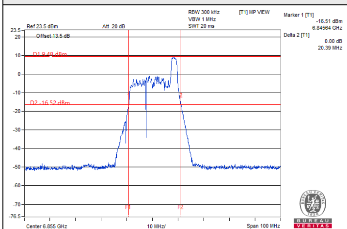
802.11be (EHT20) 26-tone RU / Chain 0 : CH 181@8
