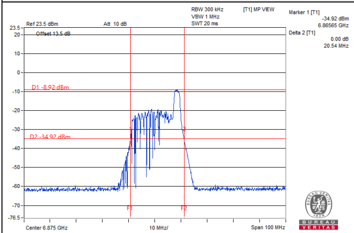
802.11be (EHT20) 26-tone RU / Chain 0 : CH 185@0
