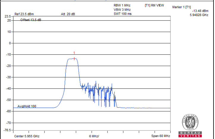
802.11be (EHT20) 52-tone RU / Chain 0 : CH 1@37
