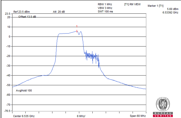
802.11be (EHT20) 106+26-tone MRU / Chain 1 : CH 117@1
