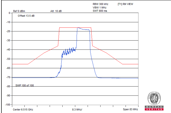
802.11be (EHT20) 106-tone RU / Chain 0 : CH 113@54
