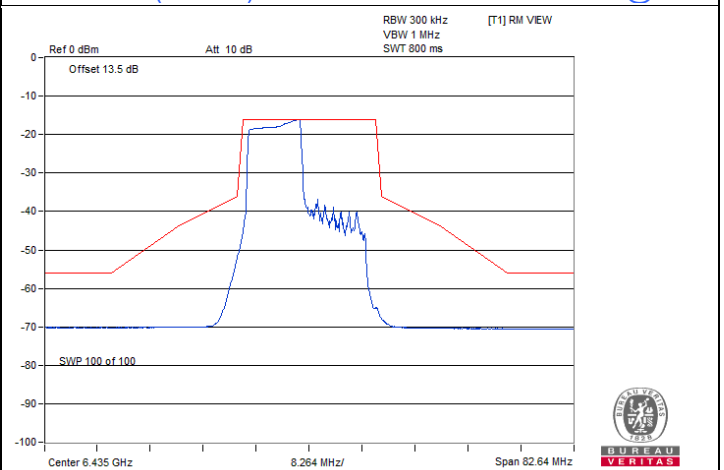
802.11be (EHT20) 106-tone RU / Chain 1 : CH 97@53
