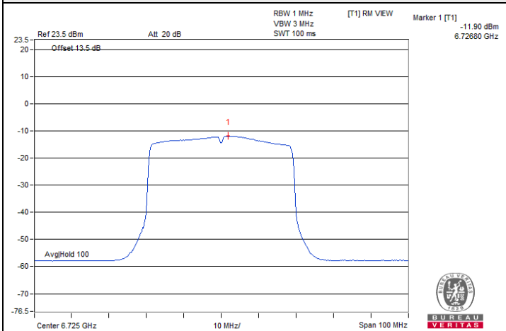
802.11be (EHT40) 484-tone RU / Chain 1 : CH 155
