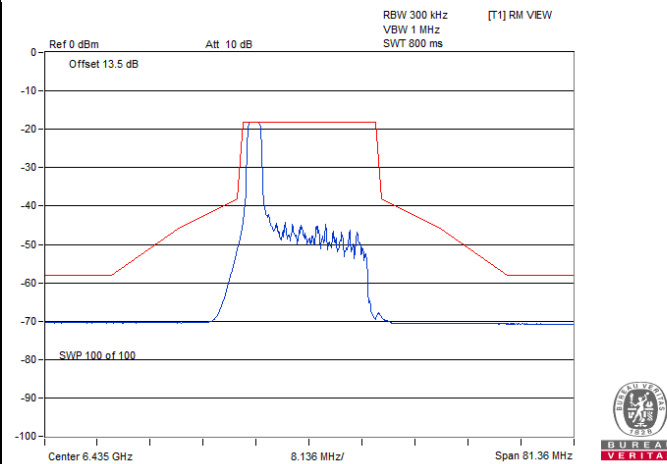
802.11be (EHT20) 26-tone RU / Chain 1 : CH 97@0
