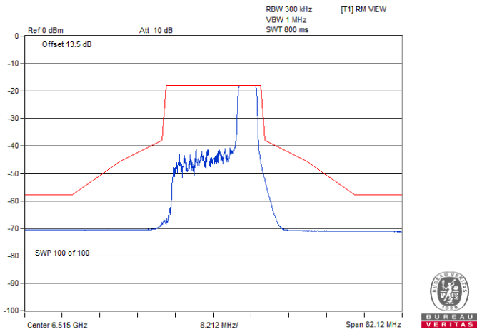
802.11be (EHT20) 52-tone RU / Chain 0 : CH 113@40
