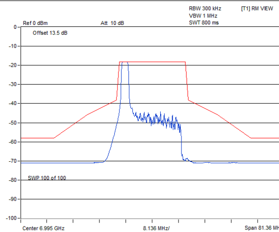
802.11be (EHT20) 26-tone RU / Chain 0 : CH 209@0
