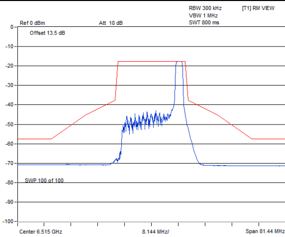
802.11be (EHT20) 26-tone RU / Chain 0 : CH 113@8
