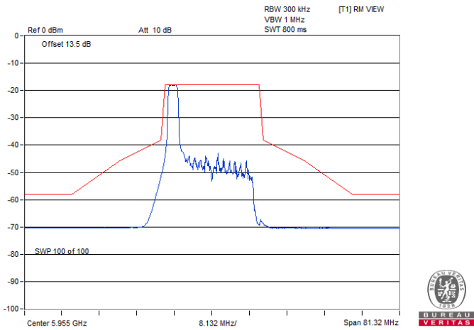
802.11be (EHT20) 26-tone RU / Chain 1 : CH 1@0
