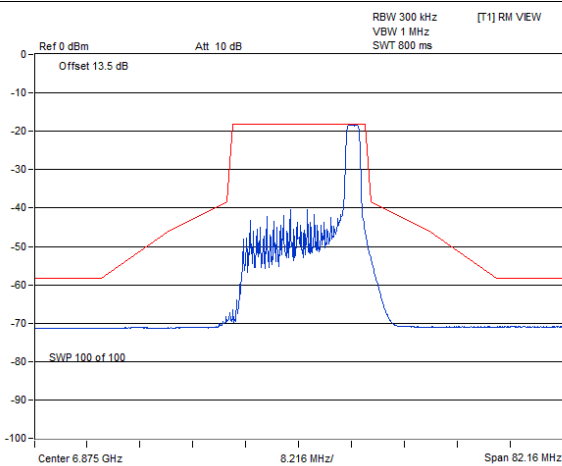
802.11be (EHT20) 26-tone RU / Chain 0 : CH 185@0
