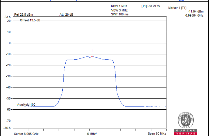
802.11be (EHT20) 242-tone RU / Chain 1 : CH 209@61
