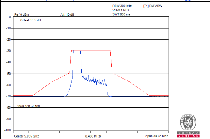
802.11be (EHT20) 52-tone RU / Chain 1 : CH 2@0
