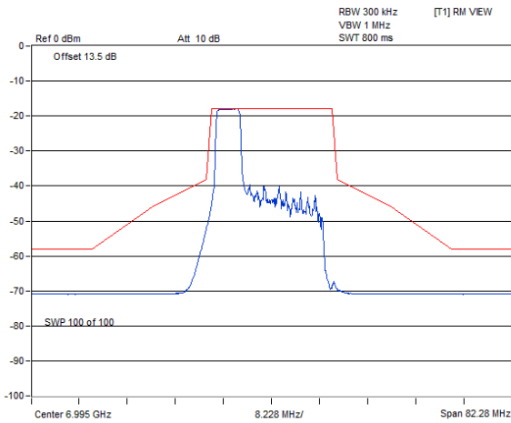
802.11be (EHT20) 52-tone RU / Chain 1 : CH 209@37
