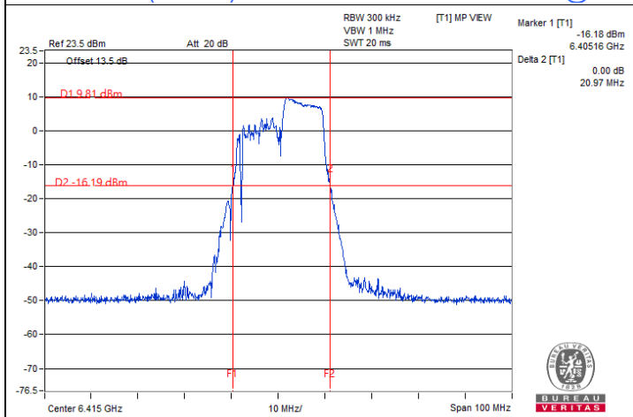
802.11be (EHT20) 106-tone RU / Chain 0 : CH 93@54
