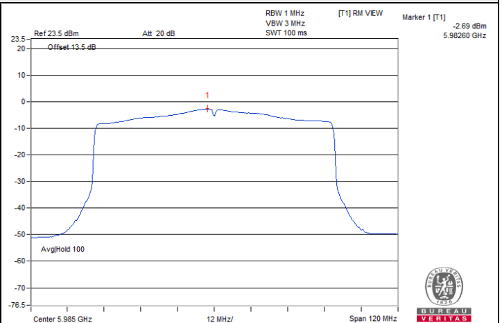
802.11be (EHT80) 996-tone RU / Chain 1 : CH 7@67
