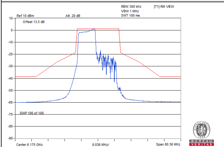
802.11be (EHT20) 106-tone RU / Chain 0 : CH 45@53
