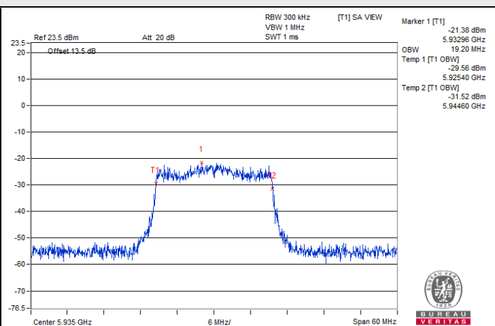
802.11be (EHT20) / Chain 1 : CH 2
