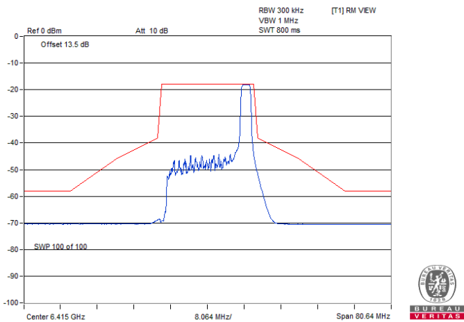
802.11be (EHT20) 26-tone RU / Chain 1 : CH 93@8
