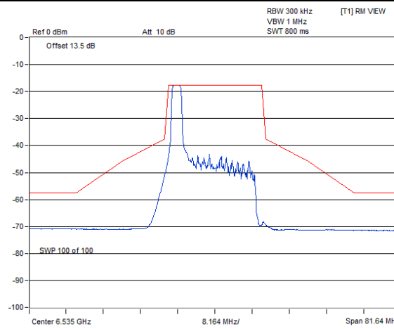
802.11be (EHT20) 26-tone RU / Chain 0 : CH 117@0
