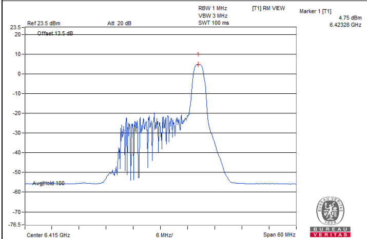
802.11be (EHT20) 26-tone RU / Chain 1 : CH 93@8
