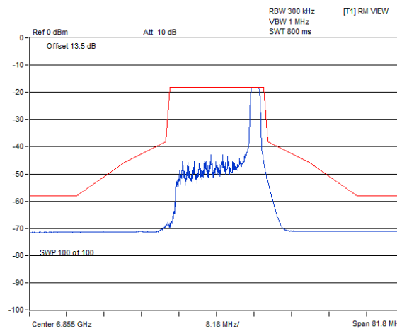
802.11be (EHT20) 26-tone RU / Chain 0 : CH 181@8
