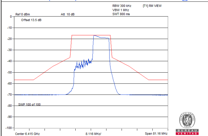
802.11be (EHT20) 106-tone RU / Chain 1 : CH 93@54
