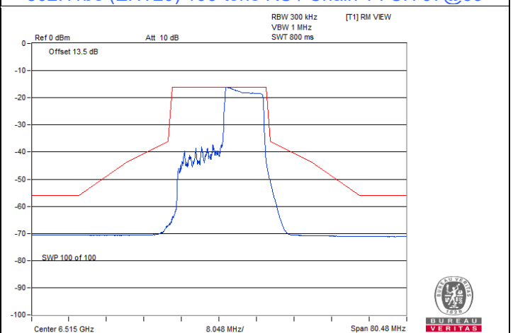
802.11be (EHT20) 106-tone RU / Chain 1 : CH 113@54
