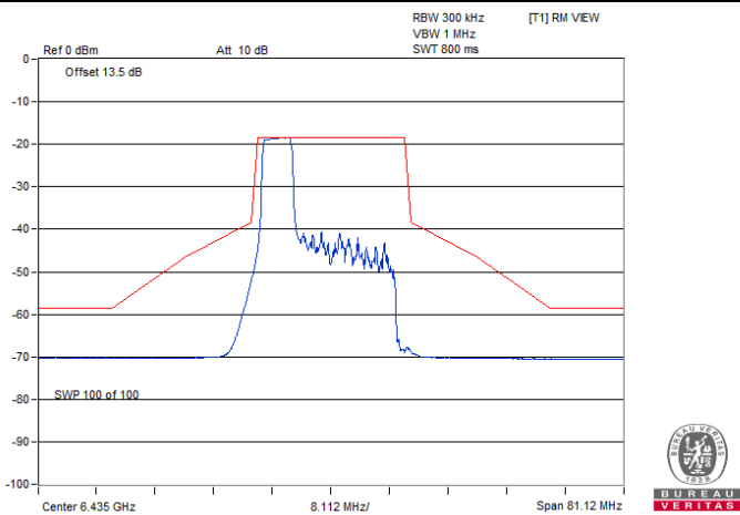
802.11be (EHT20) 52-tone RU / Chain 0 : CH 97@37
