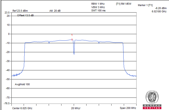
802.11be (EHT160) 2x996-tone RU / Chain 1 : CH 15
