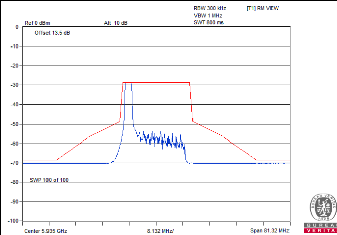
802.11be (EHT20) 26-tone RU / Chain 1 : CH 2@0
