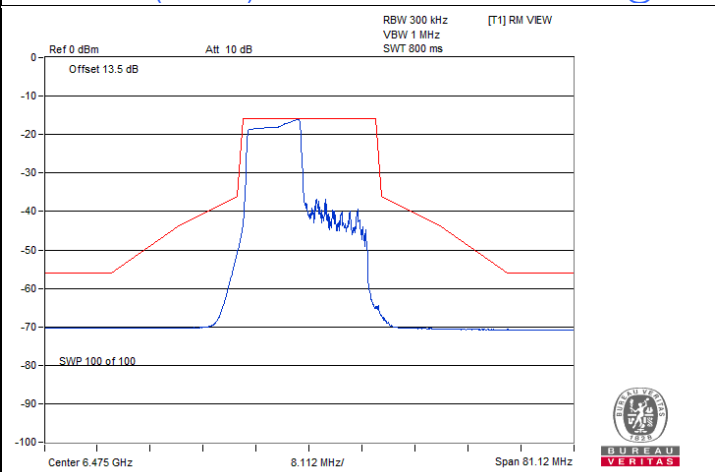
802.11be (EHT20) 106-tone RU / Chain 0 : CH 105@53
