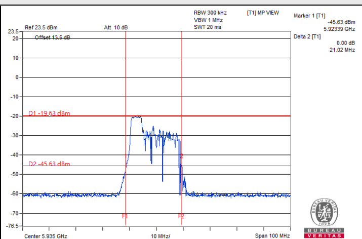
802.11be (EHT20) 52-tone RU / Chain 1 : CH 2
