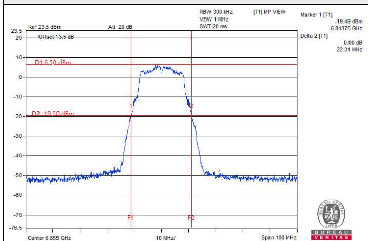
802.11a / Chain 0 : CH 181
