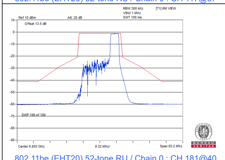
802.11be (EHT20) 52-tone RU / Chain 0 : CH 181@40
