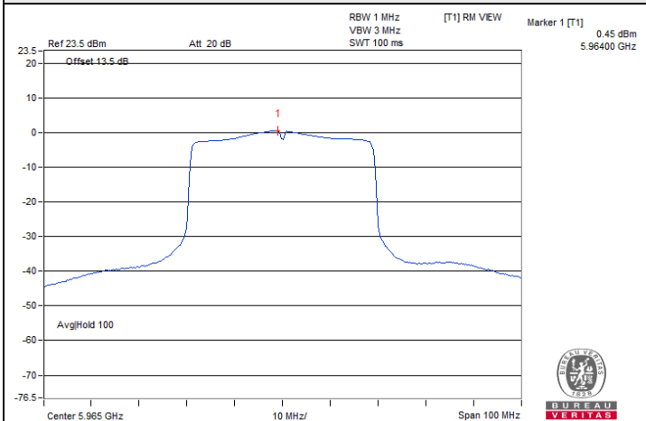
802.11be (EHT40) 484-tone RU / Chain 1 : CH 3@65
