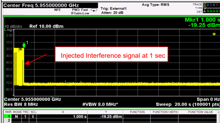
802.11be (HE20) / CH1
