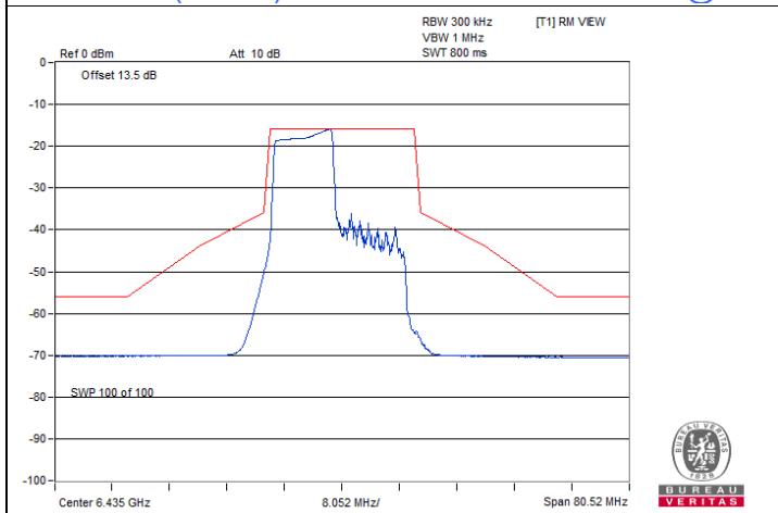
802.11be (EHT20) 106-tone RU / Chain 0 : CH 97@53
