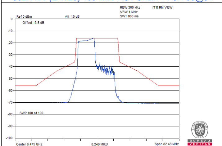
802.11be (EHT20) 106-tone RU / Chain 1 : CH 105@53
