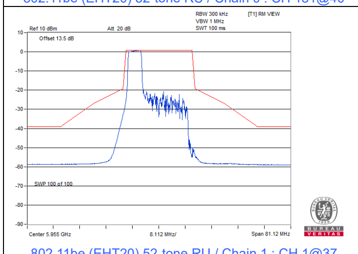
802.11be (EHT20) 52-tone RU / Chain 1 : CH 1@37
