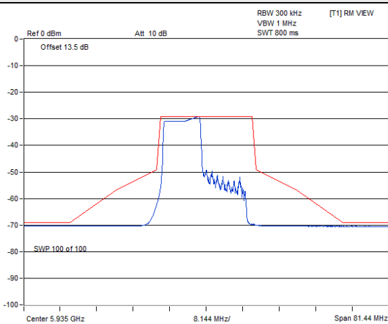
802.11be (EHT20) 106-tone RU / Chain 0 : CH 2@53
