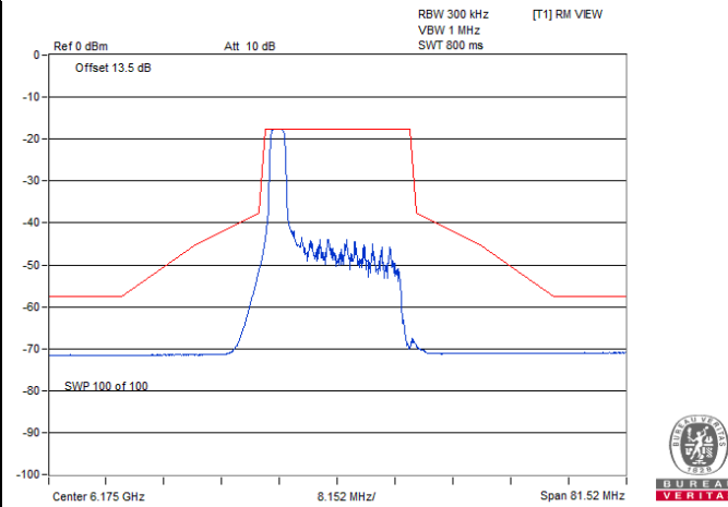
802.11be (EHT20) 26-tone RU / Chain 1 : CH 45@0
