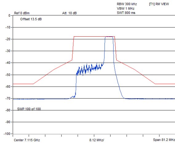
802.11be (EHT20) 52-tone RU / Chain 1 : CH 233@40
