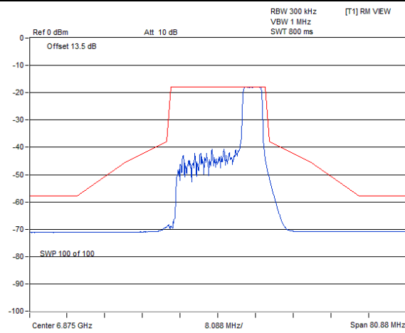
802.11be (EHT20) 52-tone RU / Chain 1 : CH 185@37
