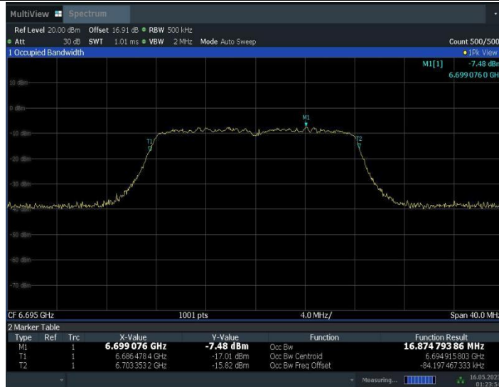
11A_Ant2_6695
