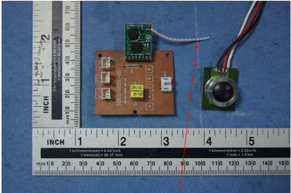
Antenna
