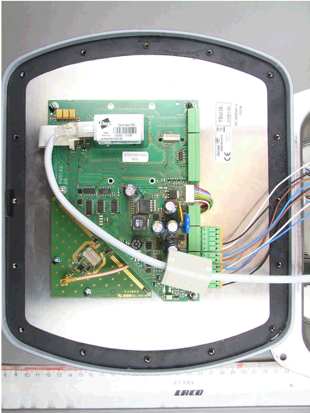
91187_d.jpg TSU25, internal top view
