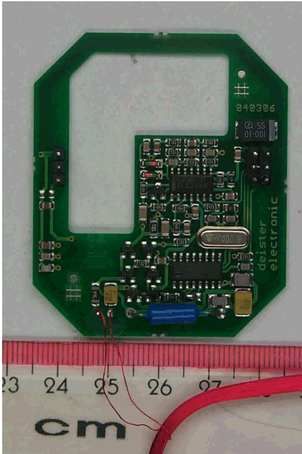
41092B_a.jpg PRD5 / SWH-4100, antenna PCB, top view
