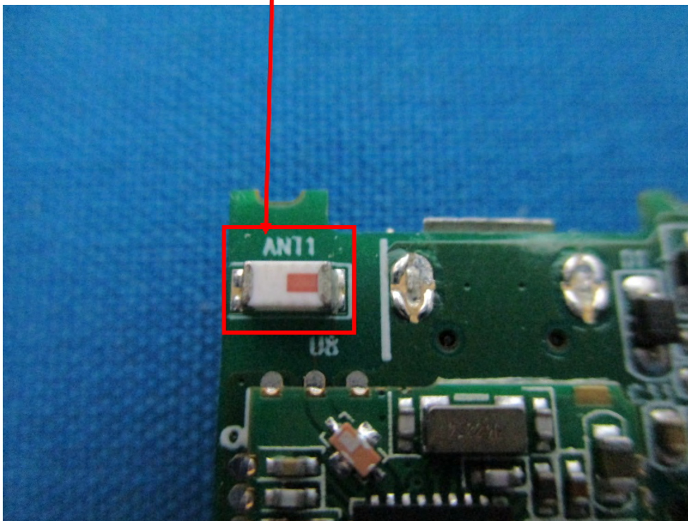
BLE Antenna – Location View
