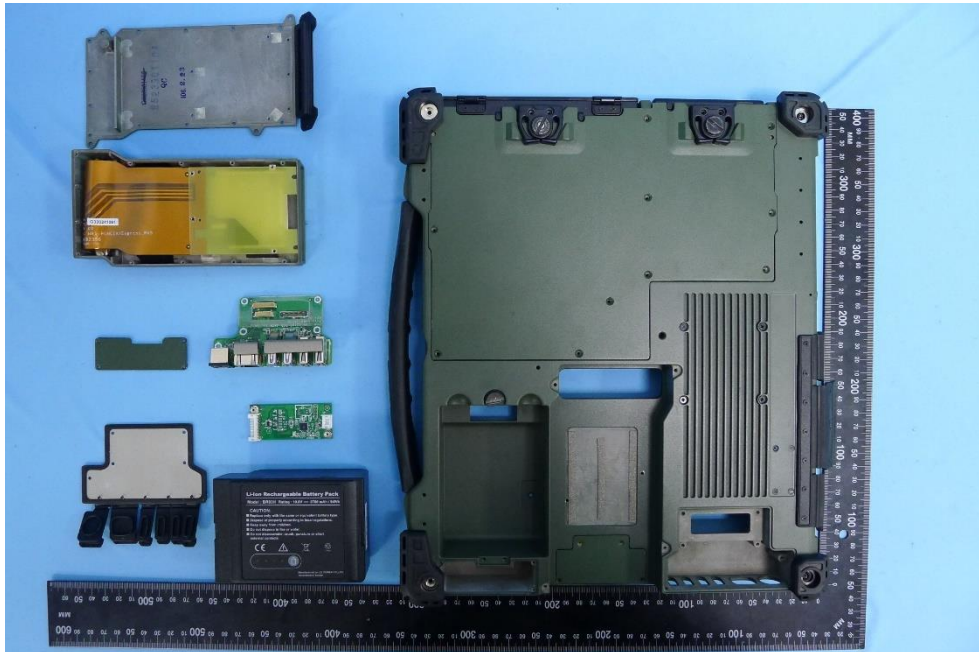
(41) EUT Photo
