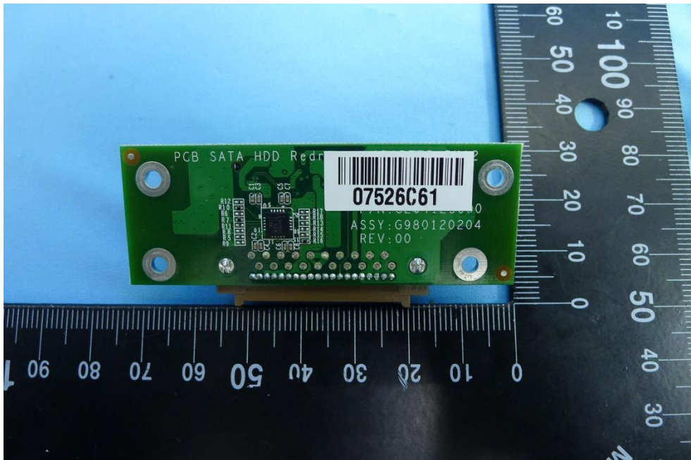
(33) EUT Photo
