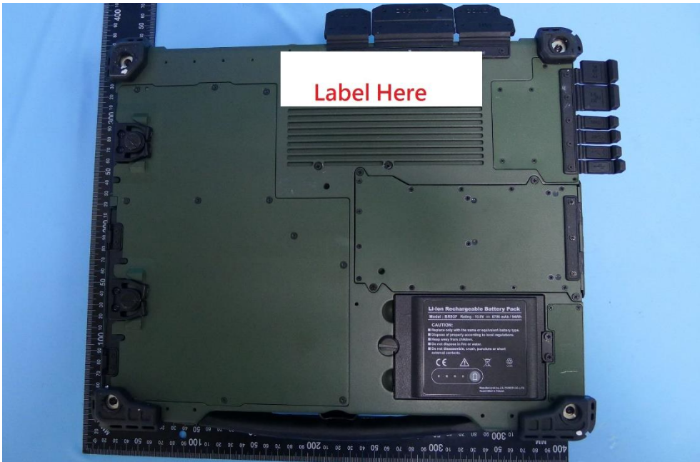
(8) EUT Photo
