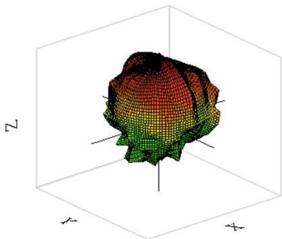
WIFI&BT 5785MHz
