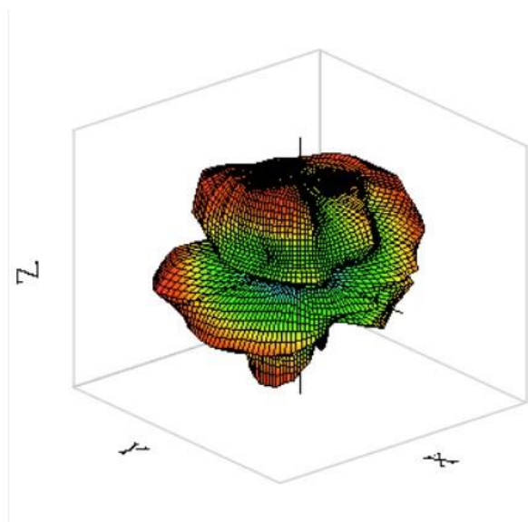
WIFI&BT 2450MHz
