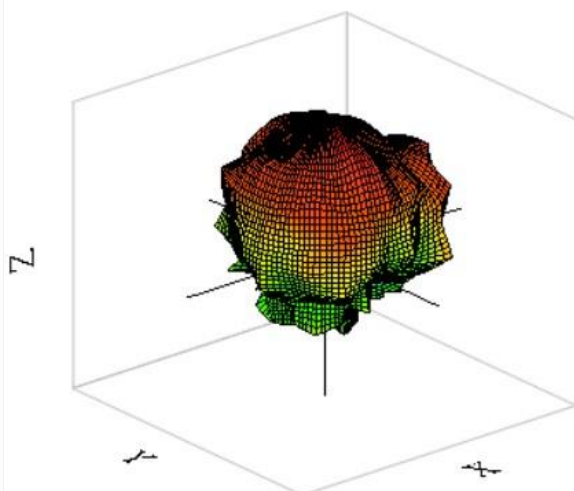
WIFI&BT 5725MHz
