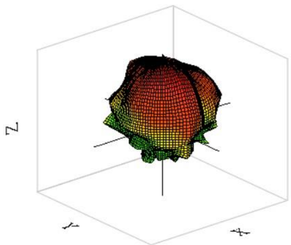
WIFI&BT 5250MHz
