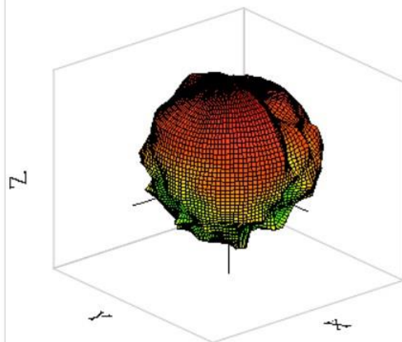
WIFI&BT 5850MHz
