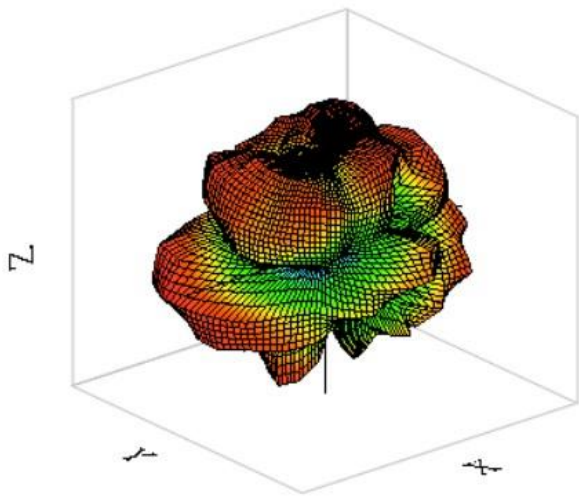
WIFI&BT 2400MHz
