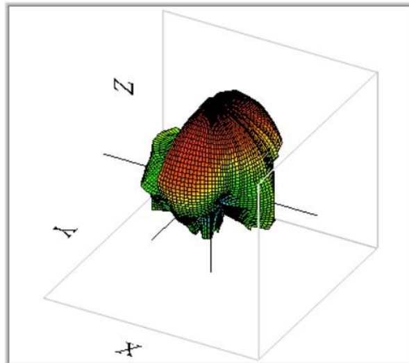
WLAN 5850MHz
