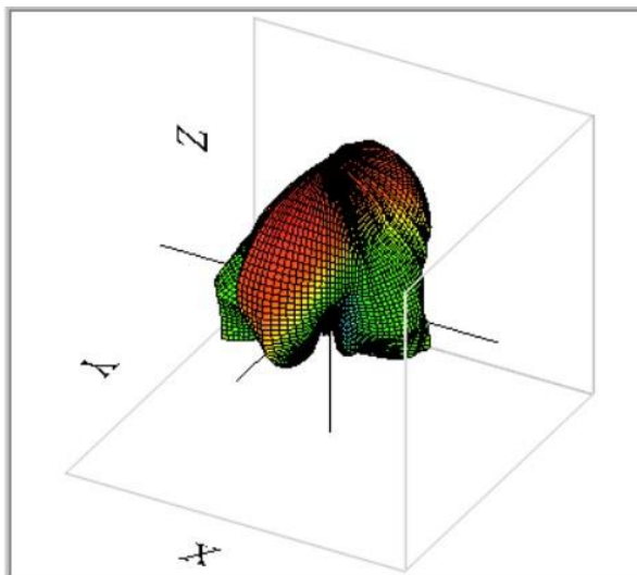
WLAN 5250MHz
