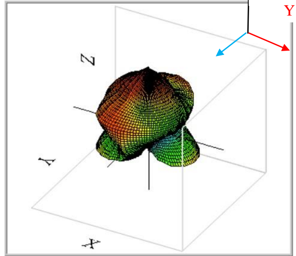
GNSS 1575MHz
