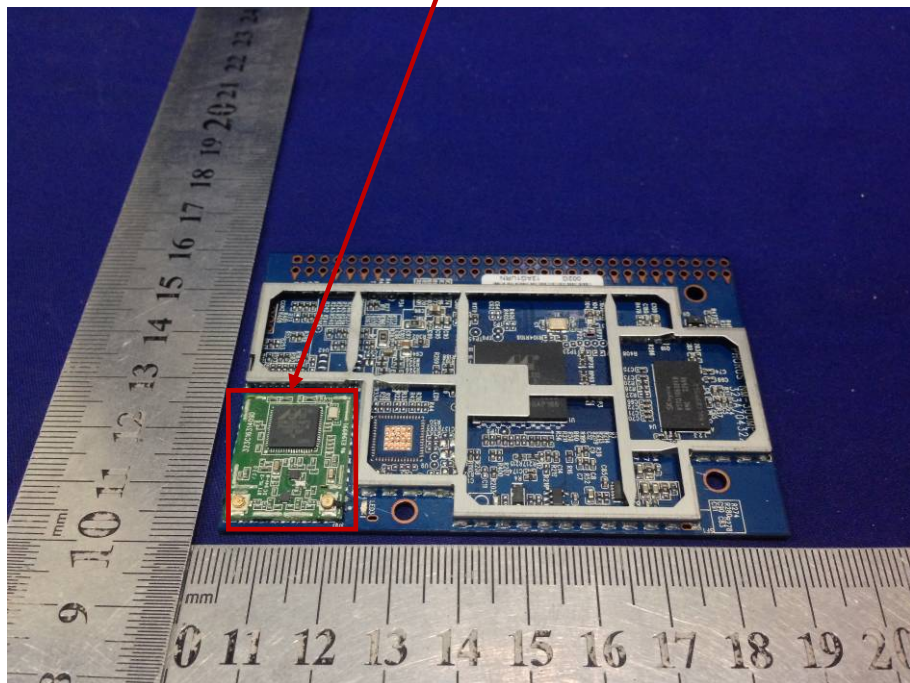
Wifi Module
