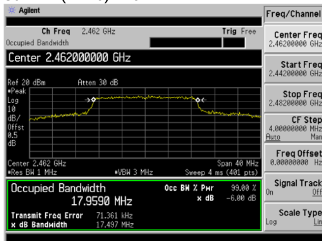
802.11n(HT20) 2462MHz
