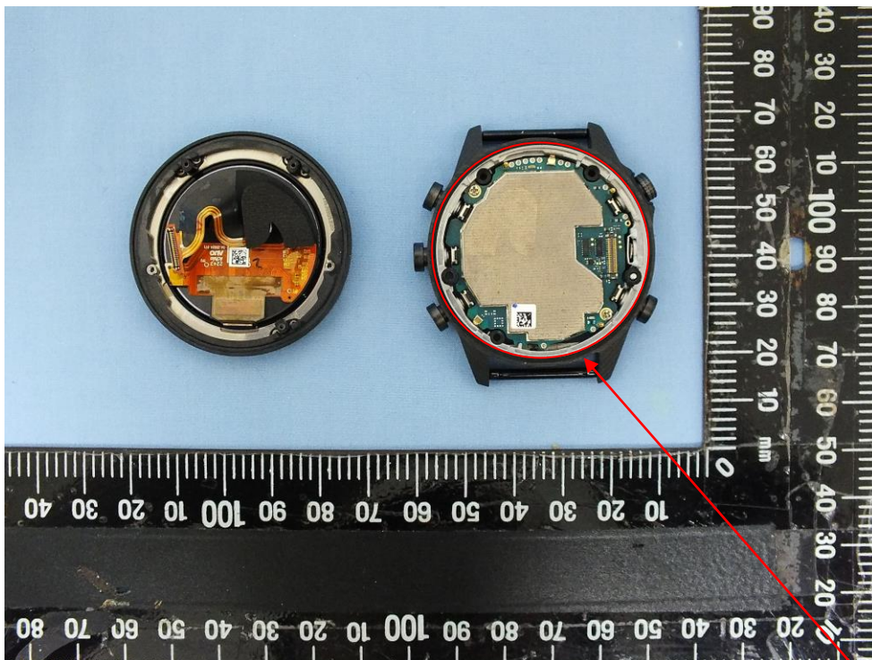
2.4GHz antenna
