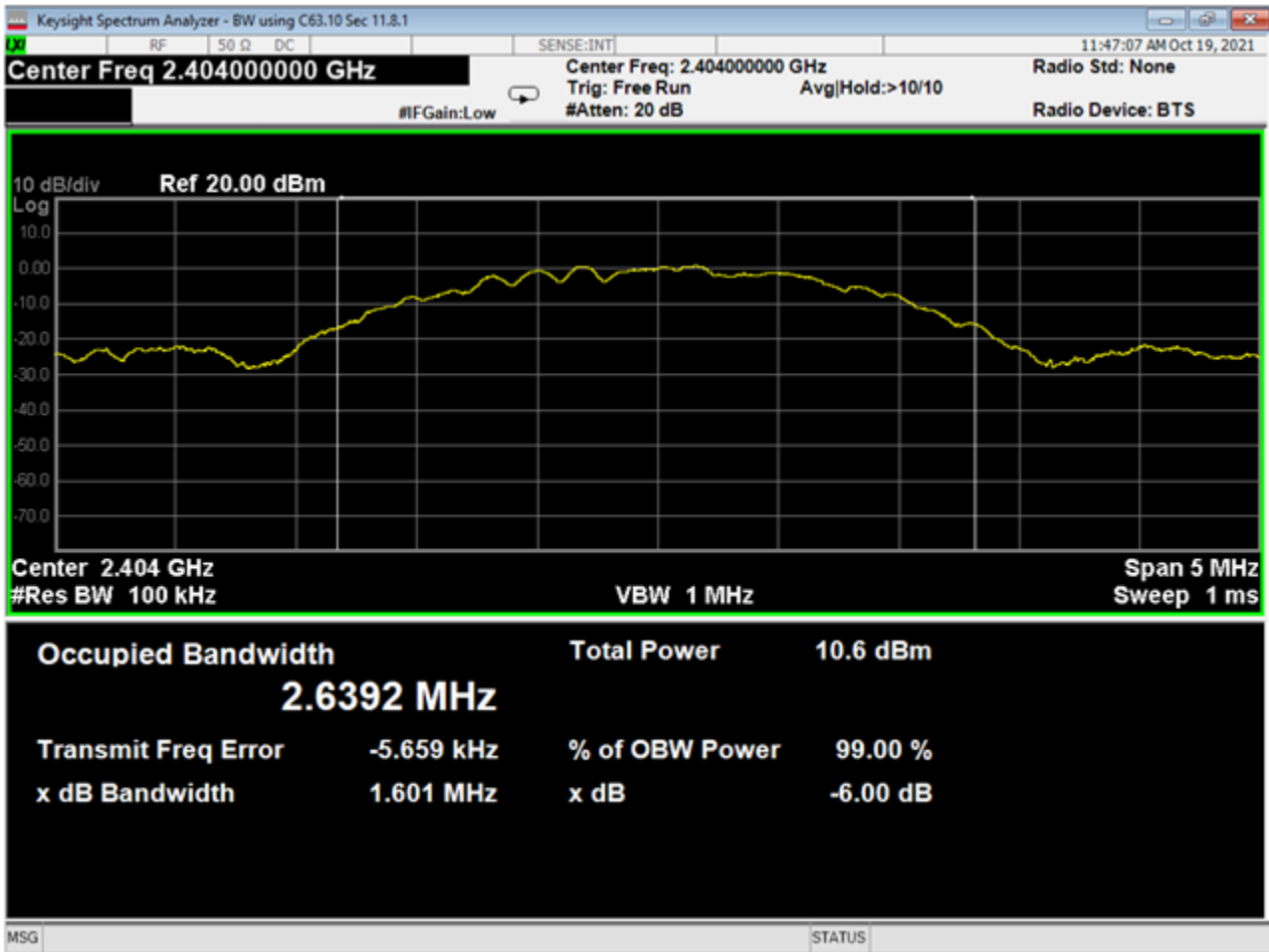
30 OBW-6dB, Low Channel, GMSK 2MB
