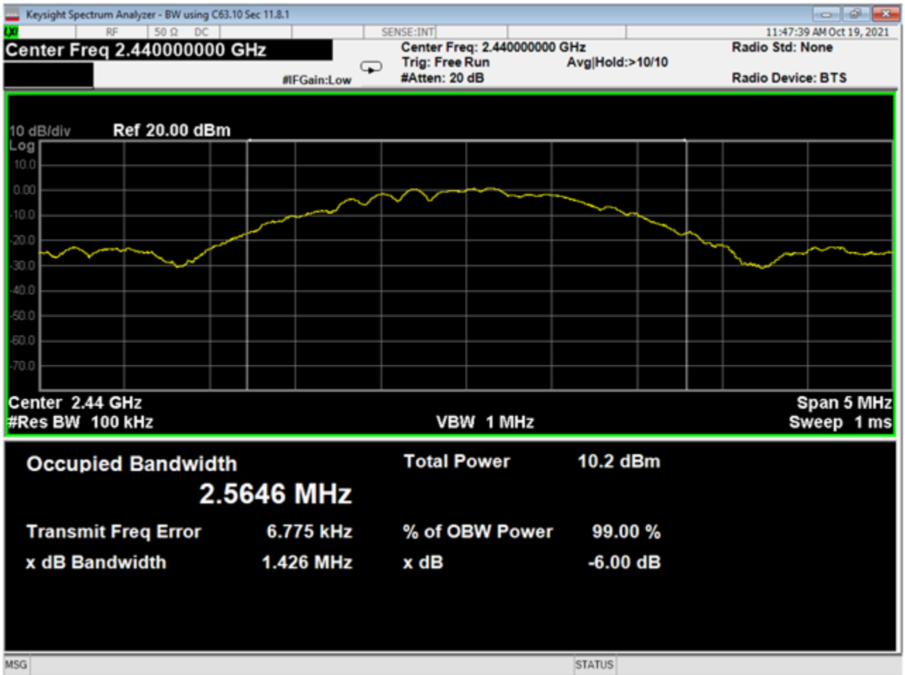
31 OBW-6dB, Mid Channel, GMSK 2MB
