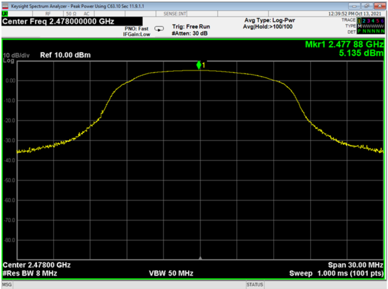
29 Power, High, BLE 2MB
