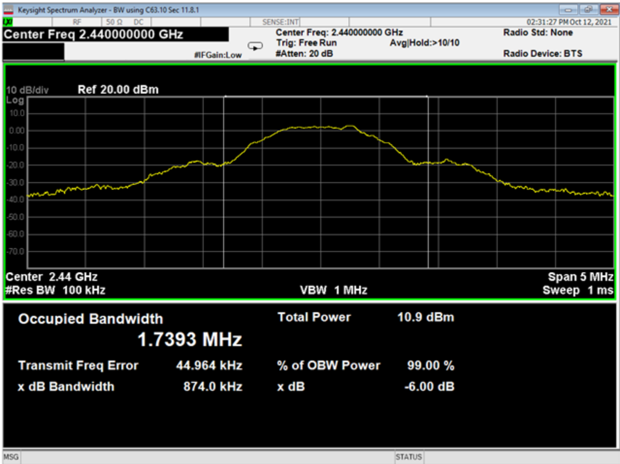
18 OBW-6dB, Mid, BLE 1MB
