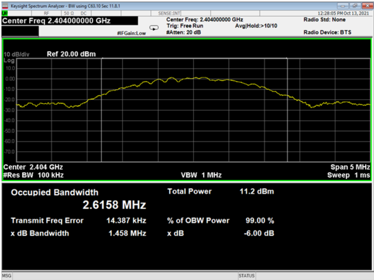
30 OBW-6dB, Low, BLE 2MB
