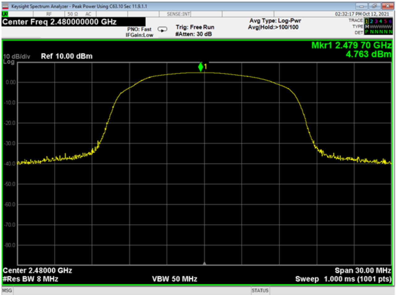
16 Power, High, BLE 1MB
