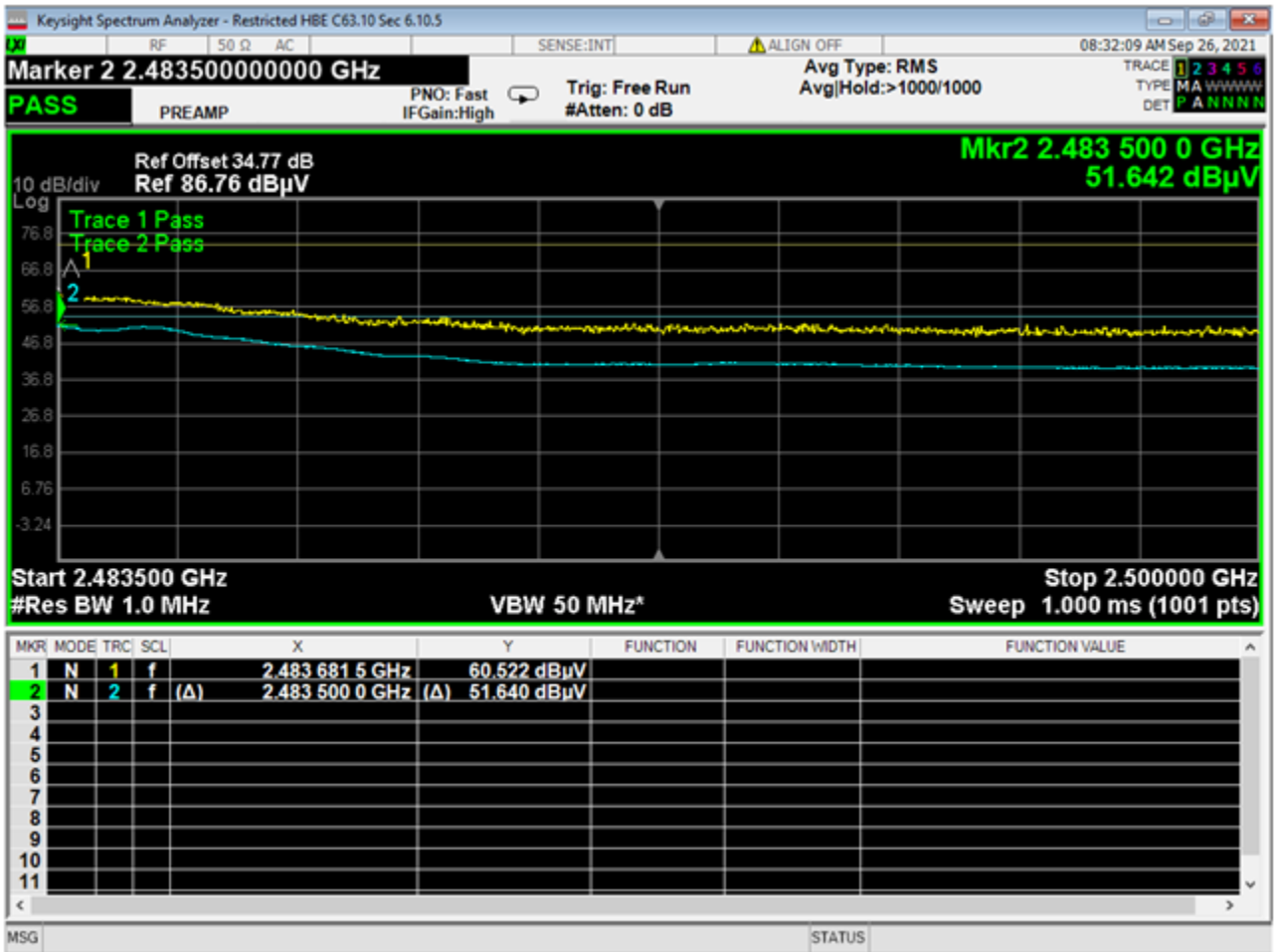
39 Higher Bandedge, Restricted, BLE 2MB
