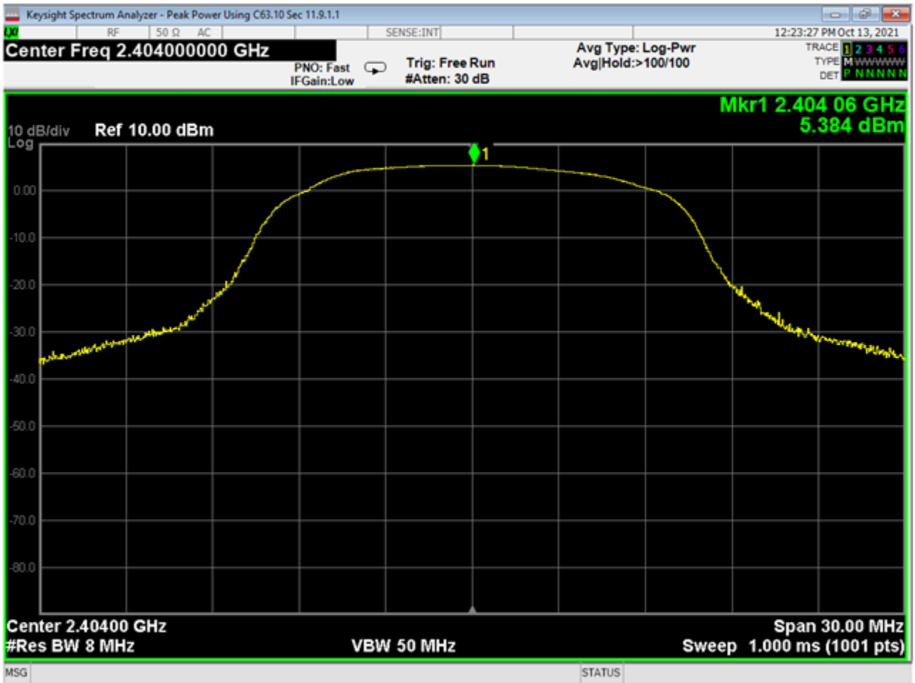
27 Power, Low, BLE 2MB
