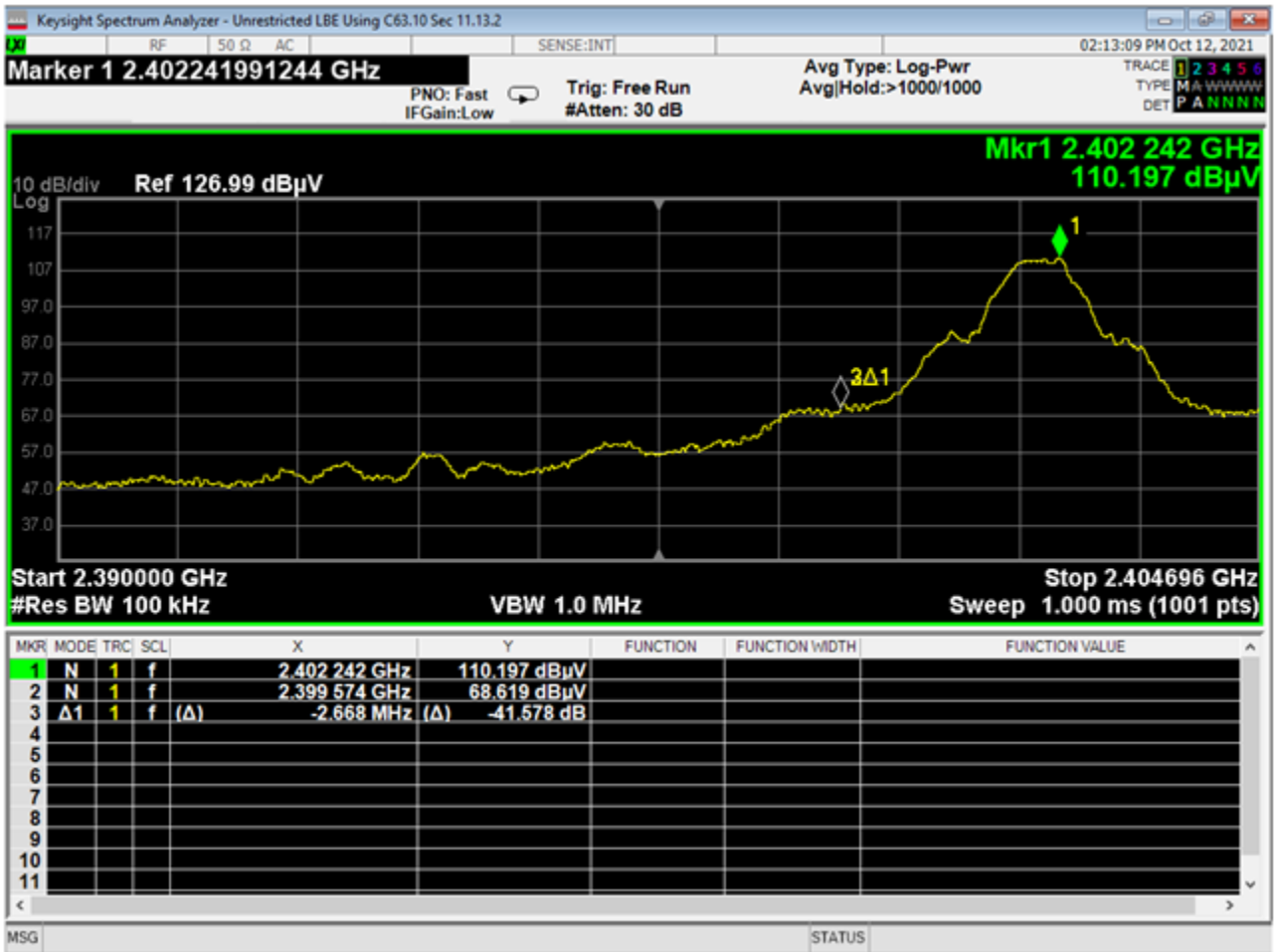
23 Lower Bandedge, Unrestricted, BLE 1MB
