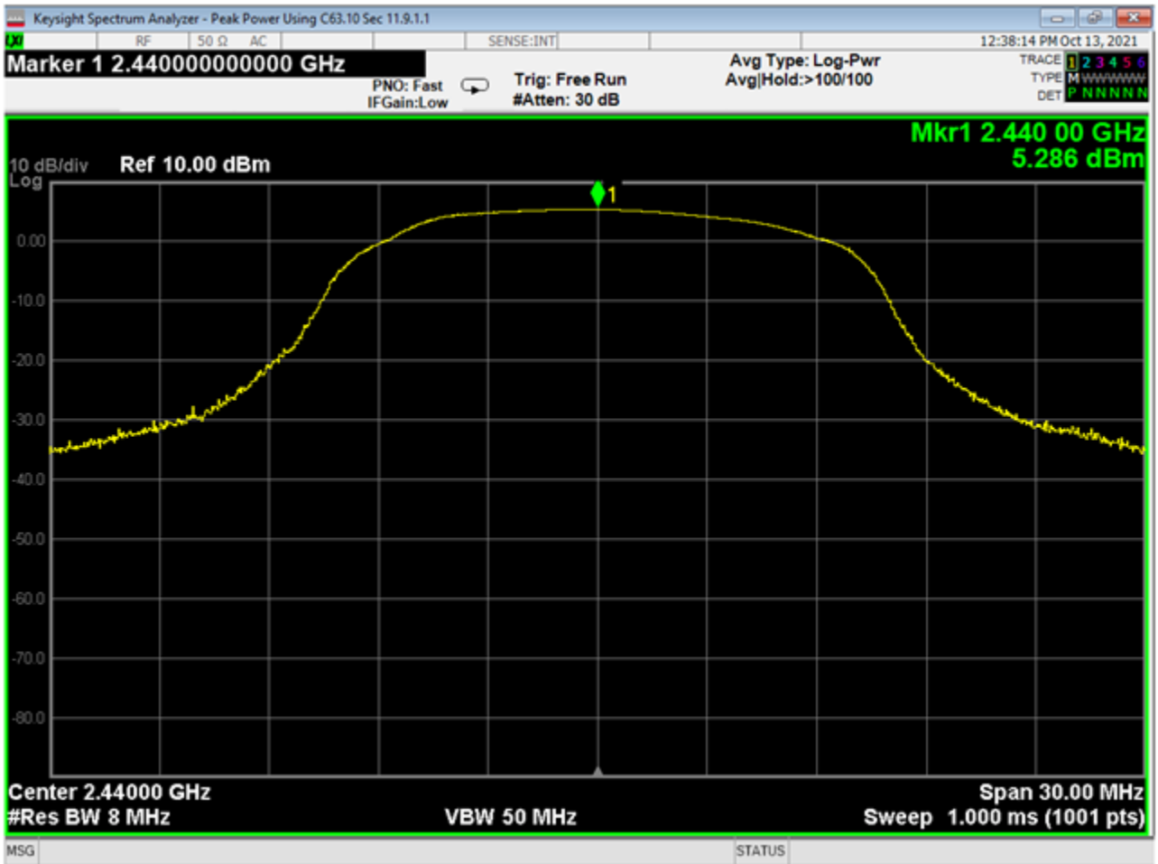
28 Power, Mid, BLE 2MB
