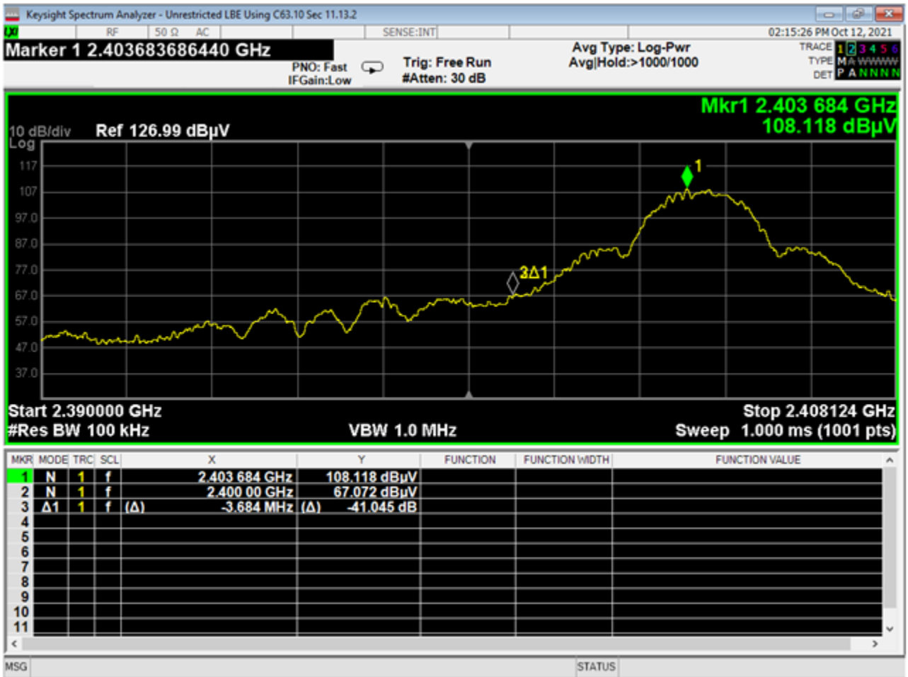
36 Lower Bandedge, Unrestricted, BLE 2MB
