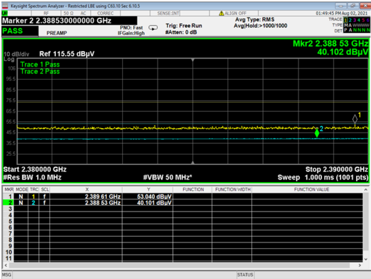
10 Lower Band Edge Restricted, 2EDR
