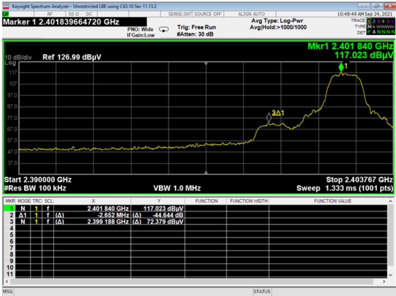
13 Lower Band Edge Unrestricted, 2EDR
