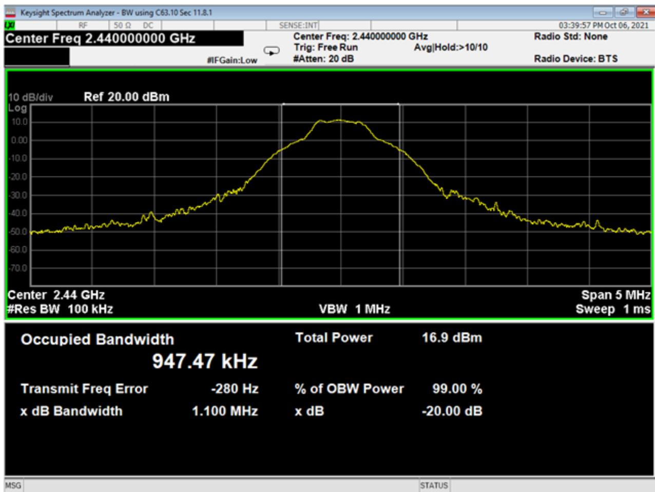
05 OBW-20dB, Mid.png
