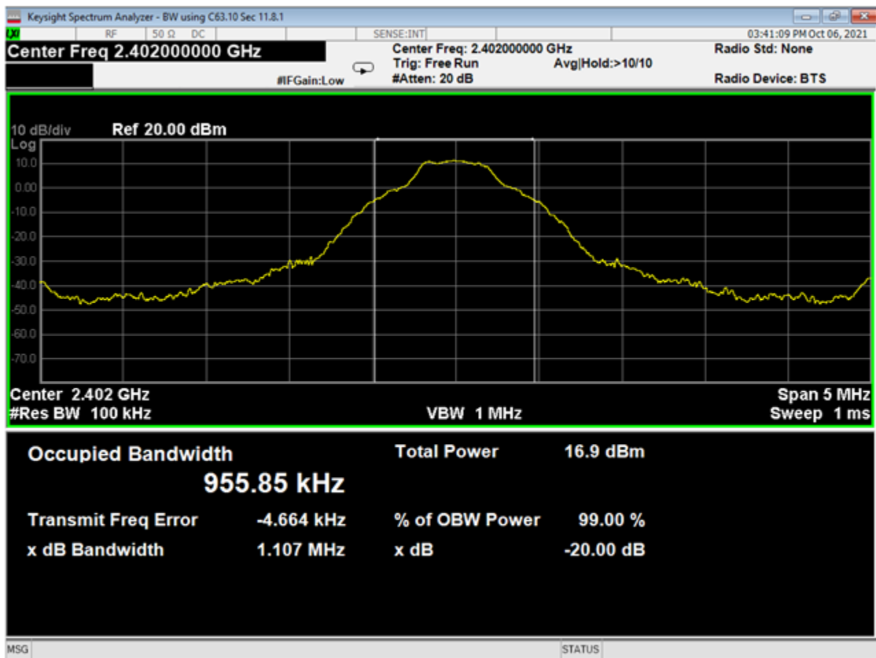
04 OBW-20dB, Low.png
