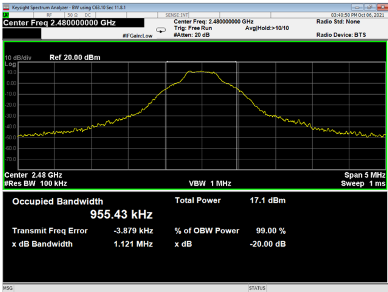
06 OBW-20dB, High.png
