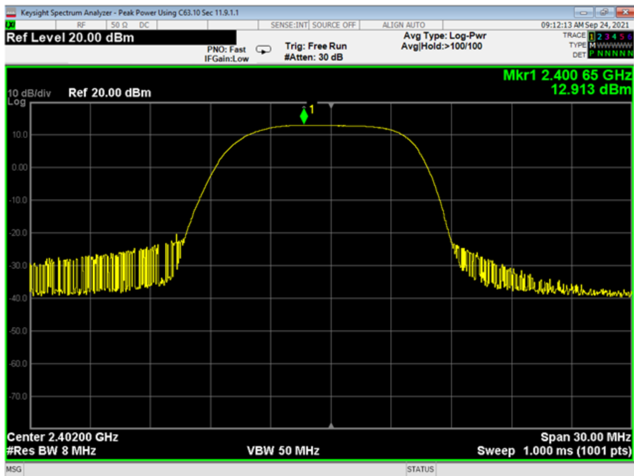
01 Pwr, Low.png
