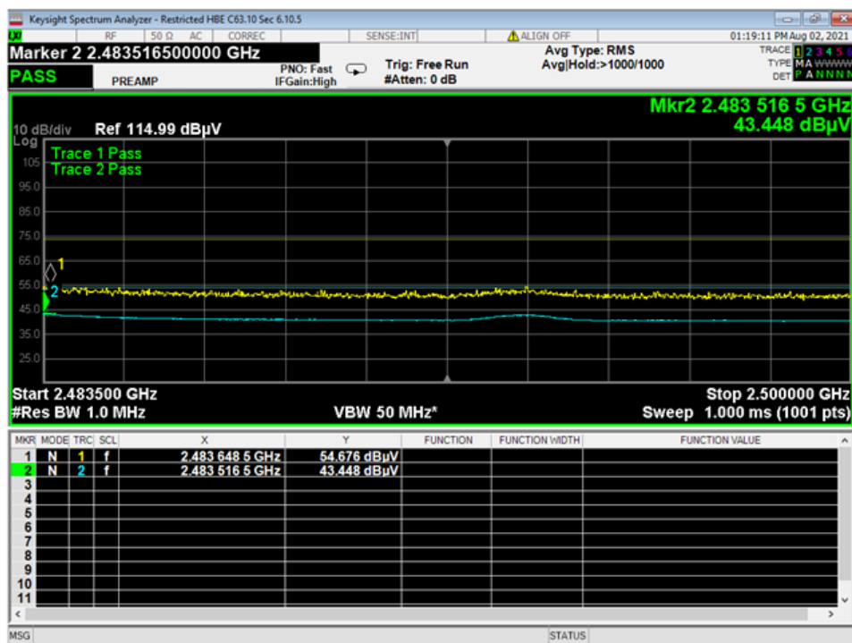
11 Higher Band Edge Restricted, 2EDR
