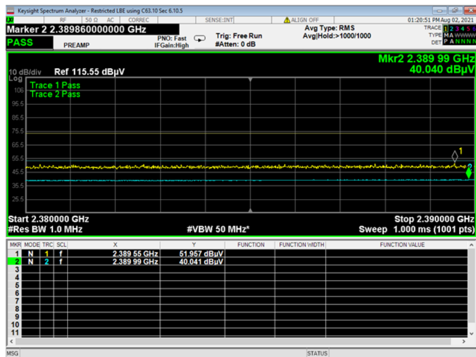
10 Lower Band Edge Restricted, 2EDR
