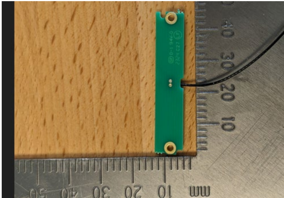
Antenna: (ANT/WiFi/BLE)
