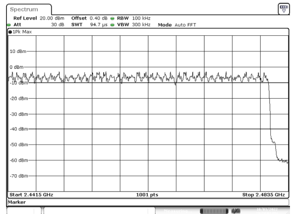
2480 MHz
