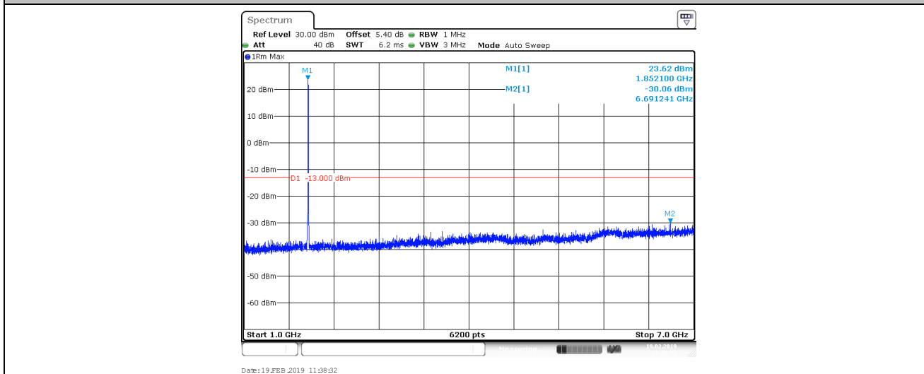
Band II_9262
