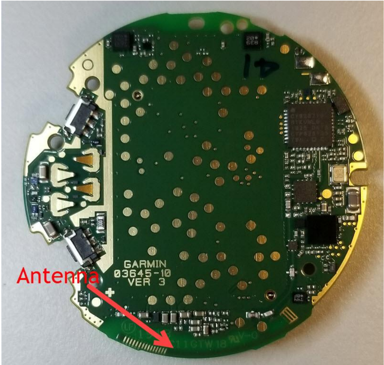
2.4 GHz antenna
