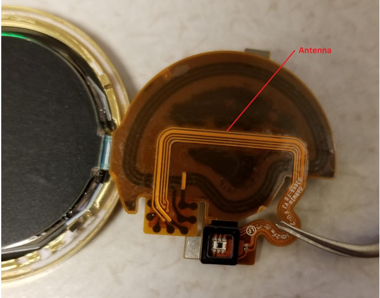
NFC Antenna
