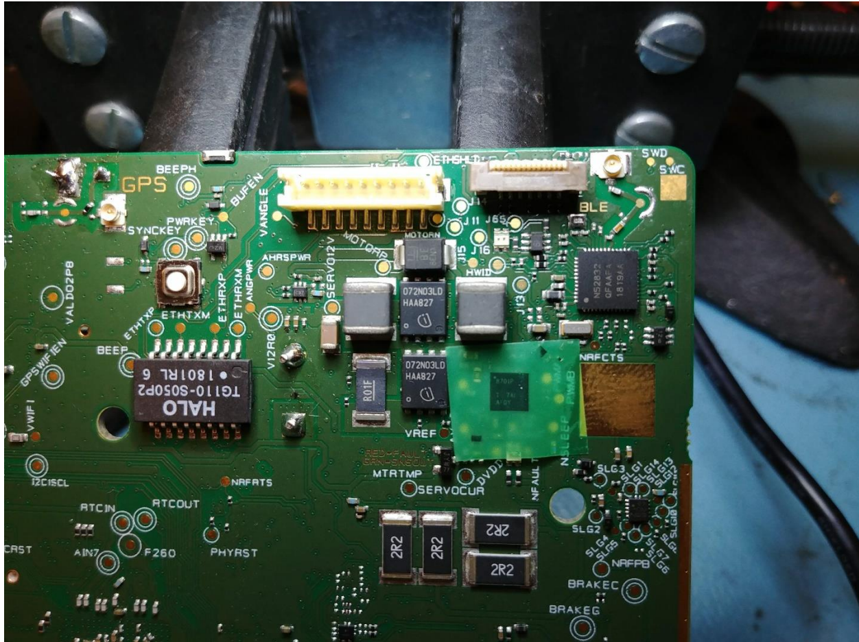
BLE radio section
