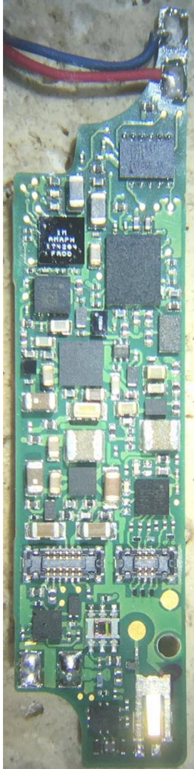
PCB top
