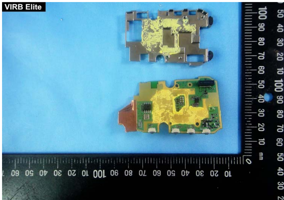
EUT Photo 8 )
