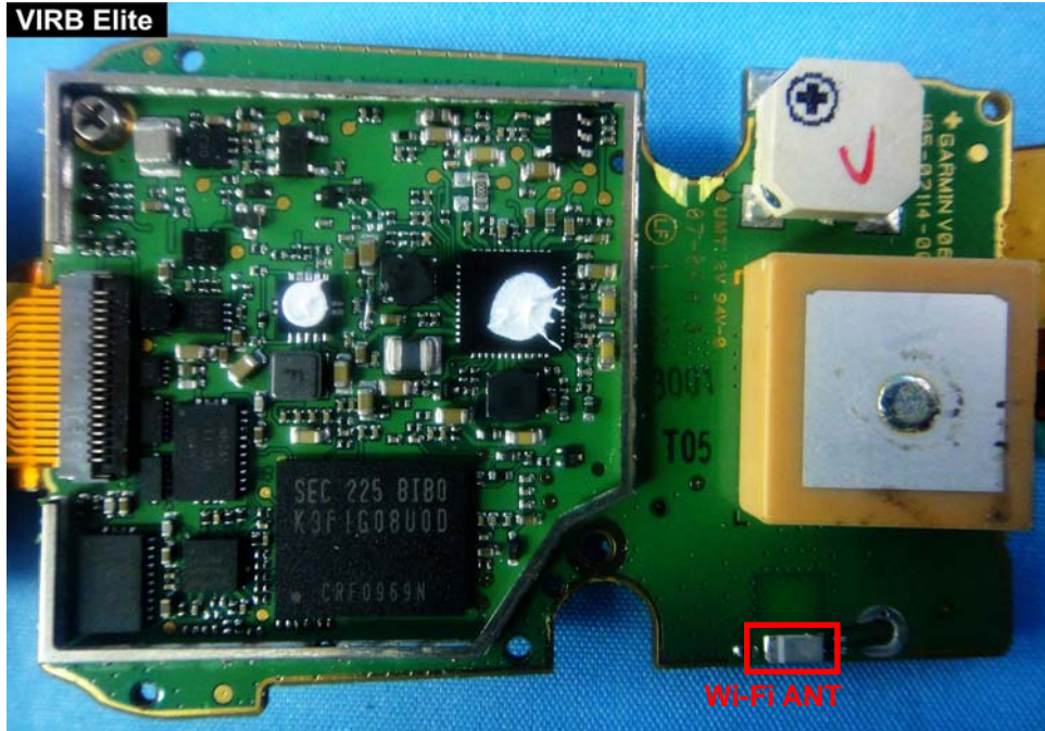
EUT Photo 13 )
