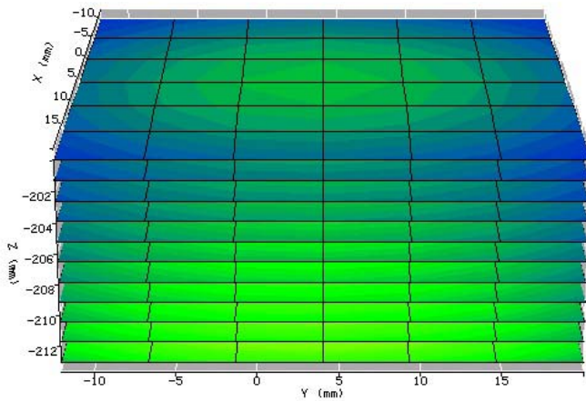
10 20 30 40 50 60 70 80 Eeff (V/m)
