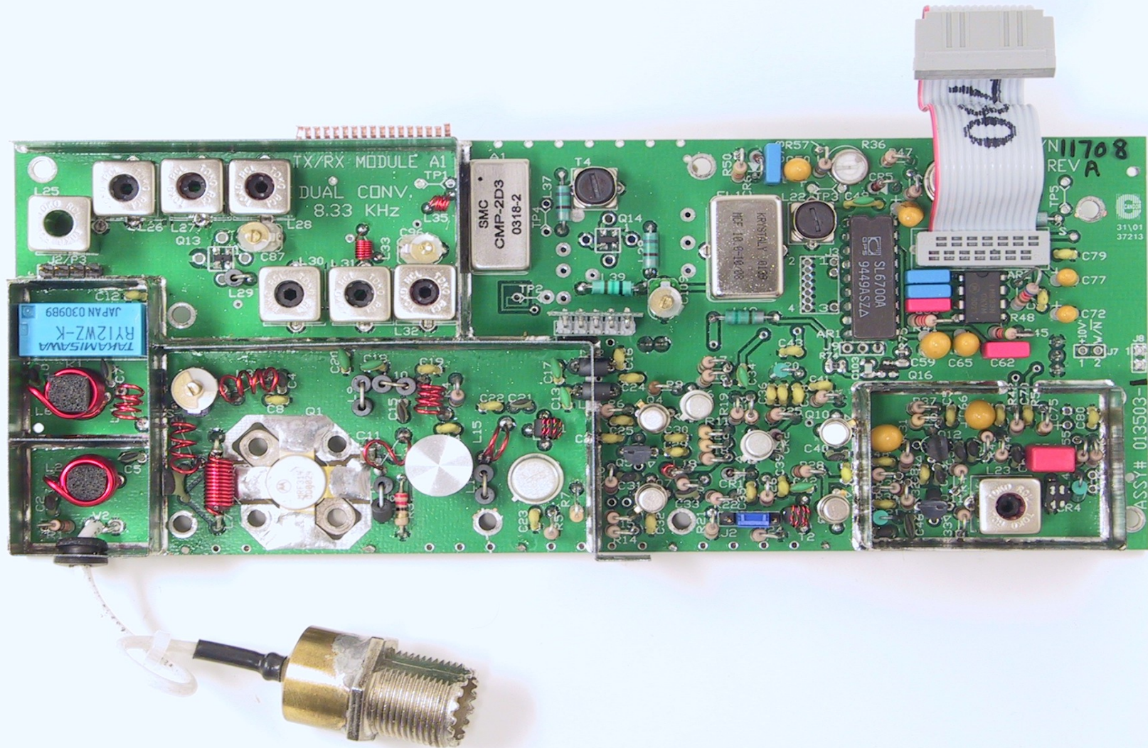
TX RX Module
