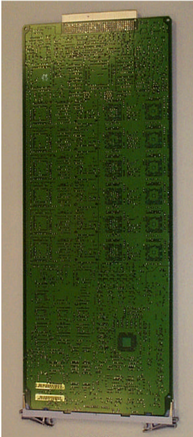
IHET6YZ1 SC4812ET 1.9 GHz MCC x 24E Back
