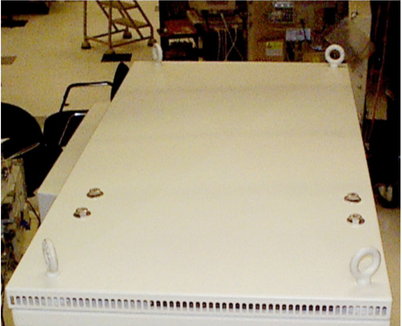
IHET6BM1 SC4812ET 1.9GHz TopView
