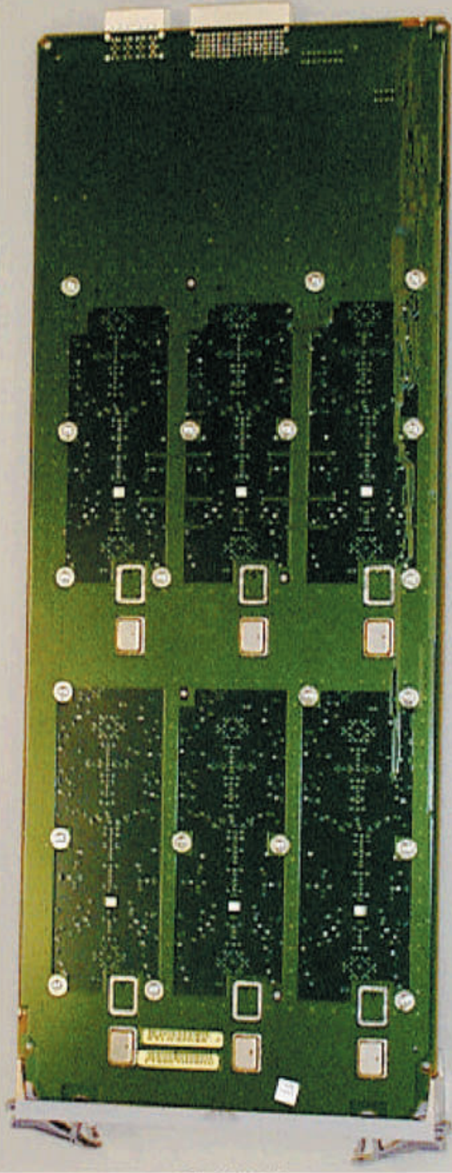
IHET6AP1 SC4812ET 1.9 GHz MPC Back
