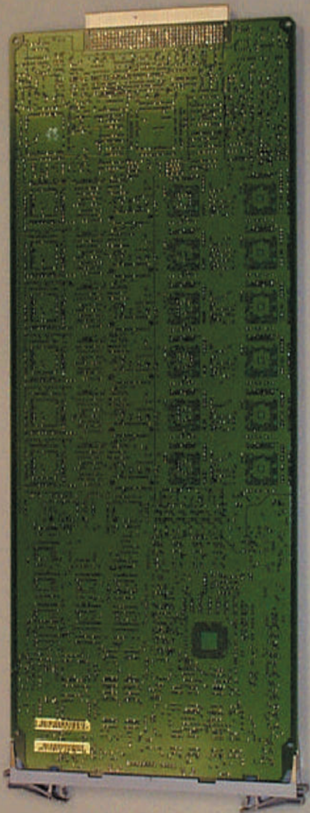
ITHET6AP1 SC4812ET 1.9 GHz MCC x 24E Back
