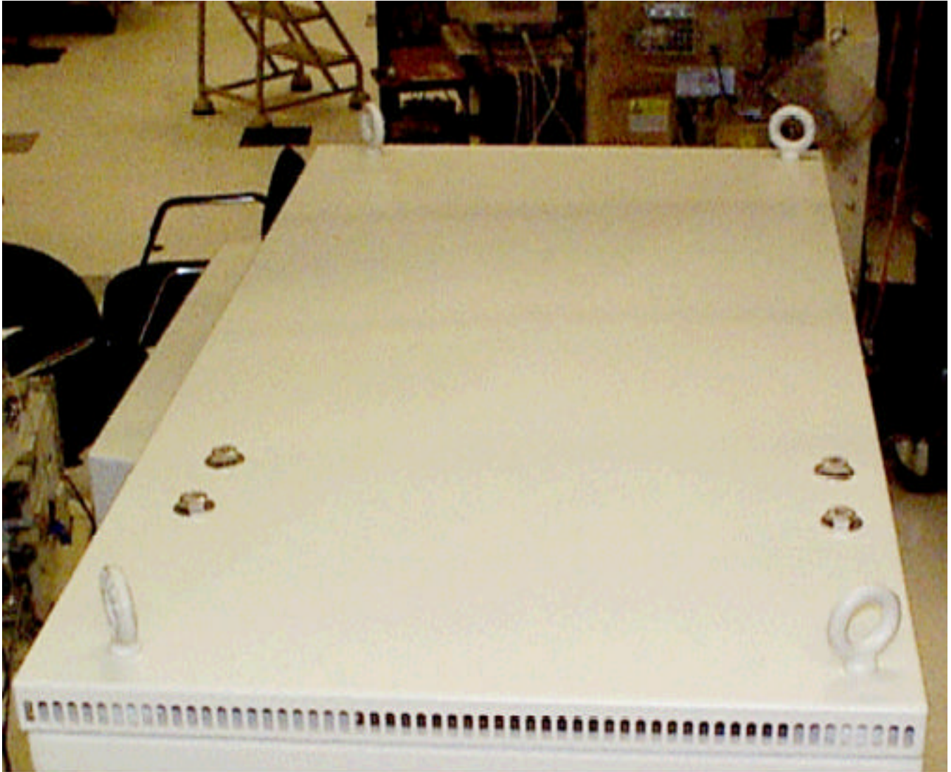
IHETSZR1 SC4812ET 800 MHz Top View
