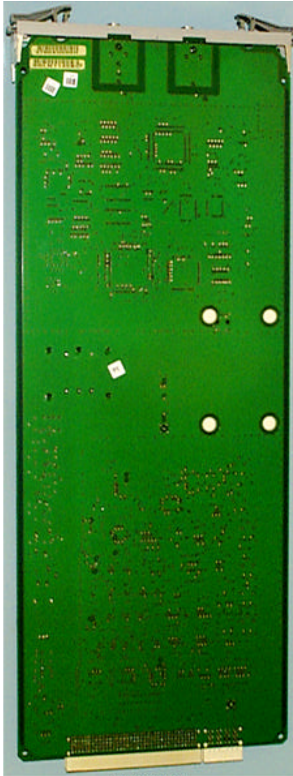
IHET5AW1 -48V SC4812T 800MHz CSM1 Back
