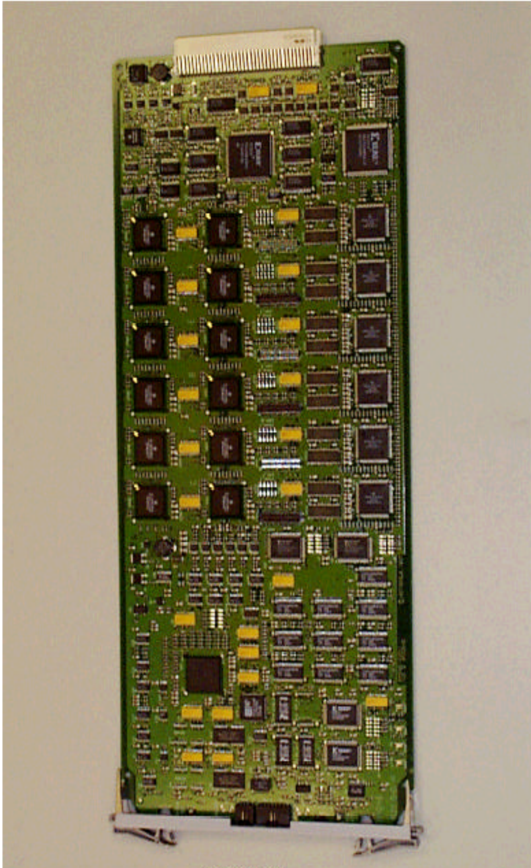
IHET5AW1 -48V SC4812T 800MHz MCC X 24E Front
