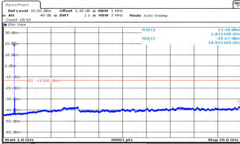
Band2-20MHz-64QAM-18900-1RB#0-Range2:1000~20000MHz
