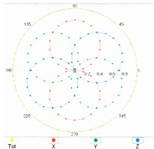
f=1800 MHz,R22
