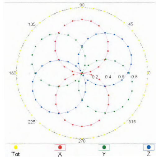
f=1800 MHz,R22
