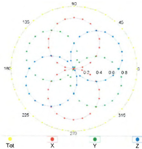
f=1800 MHz,R22
