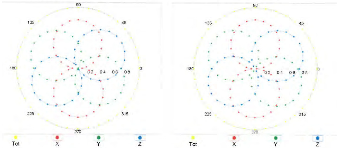
f=1800 MHz,R22
