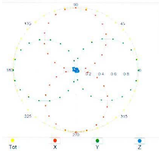
f=600 MHz, TEM, 0^\circ
