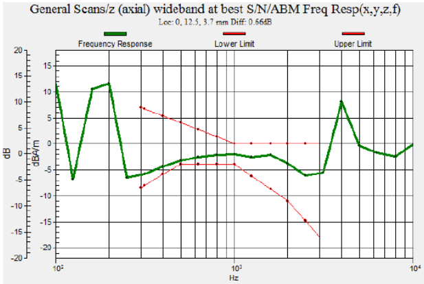
Fig 7.1 GSM850 Ch189
