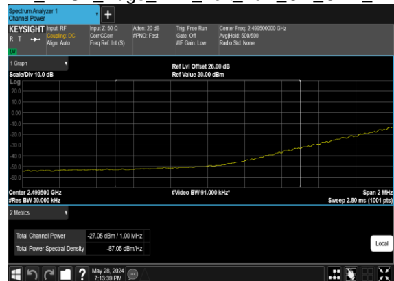
B2_N7(50M)_DFT-s-OFDM_BPSK_Edge_1RB_Left_Low_CH_CHP_PASS
